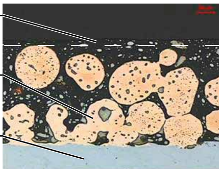
Fig. 15: Layer system
