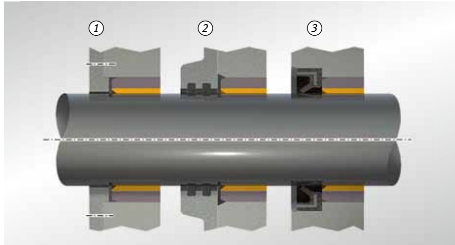
Fig. 43: Seals
