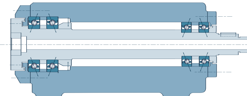
Ejemplo 4: Rodamientos MachLine MLE
