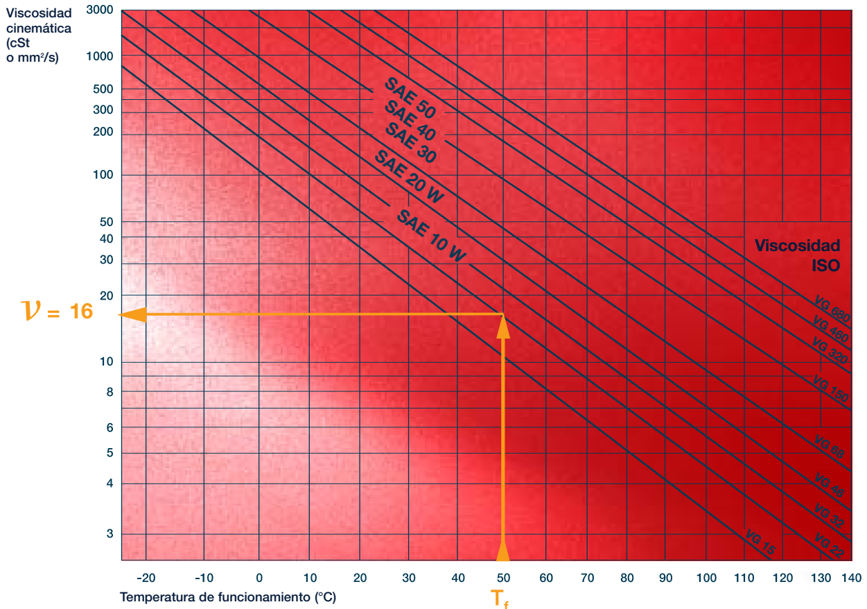
Diagrama 1: Viscosidad-temperatura
