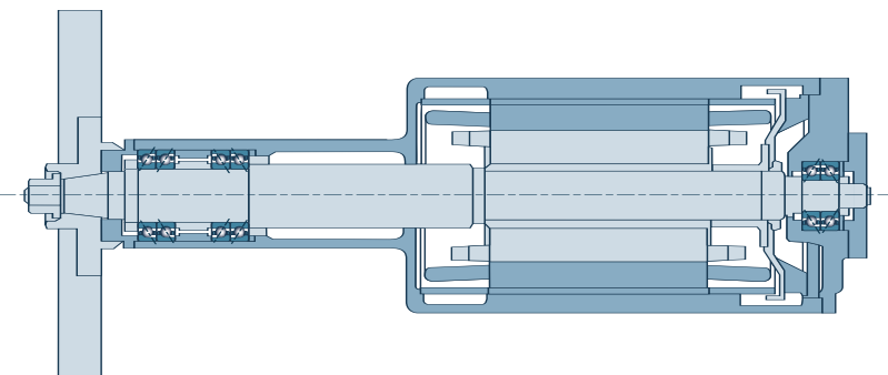
Ejemplo 5: Rodamientos MachLine Estándar
