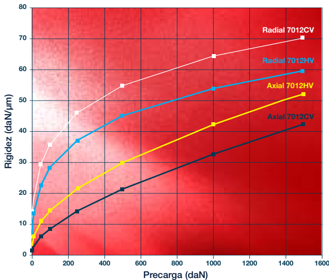
Ejemplo de un rodamiento 7012 montado en DB
