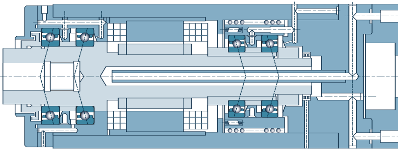
Ejemplo 2: Rodamientos MachLine ML
