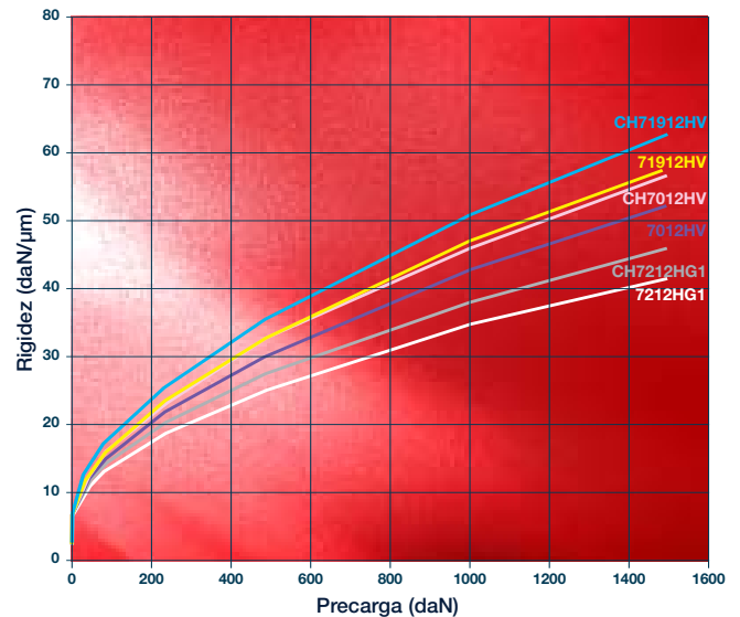
Comparativa de rigidez en función de la serie
