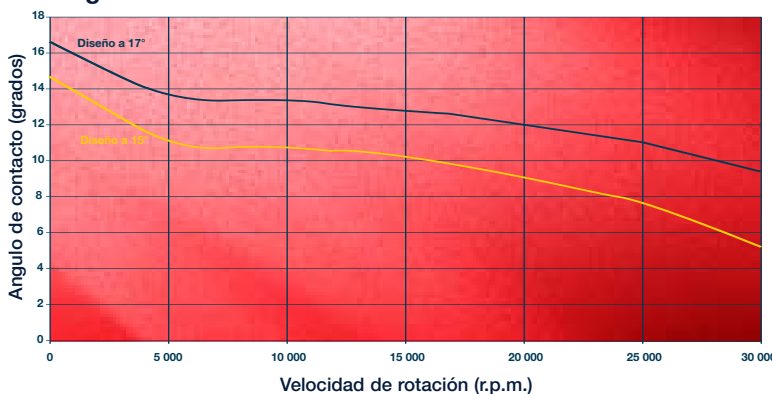
Ángulo de contacto medio teórico residual
